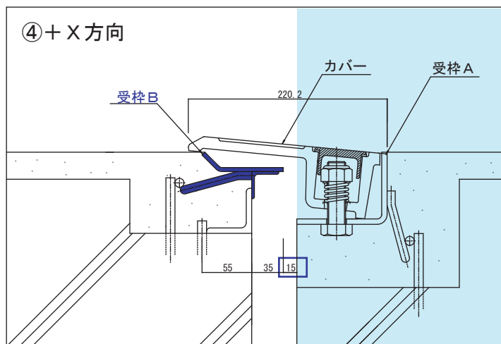
新仕様 (JX-HE-25 100-50)
