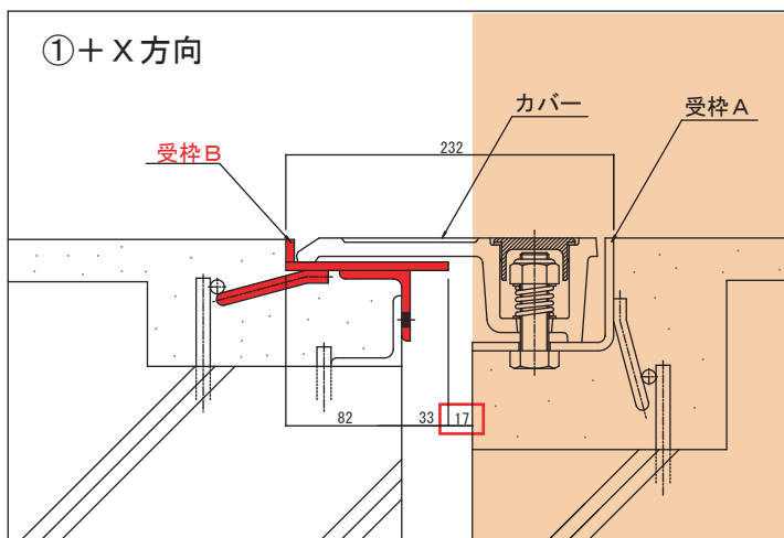
旧仕様 (HEX77-50)
