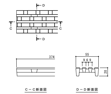
スリット蓋 詳細図 S=1:2
