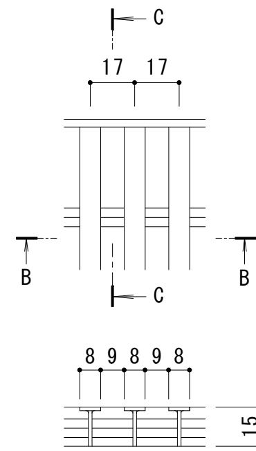
B-B断面図
