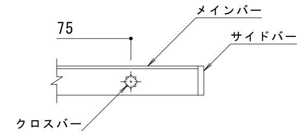
C-C断面図
