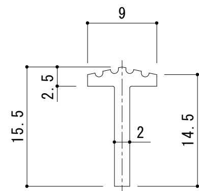
メンバー断面 S = 2 : 1
