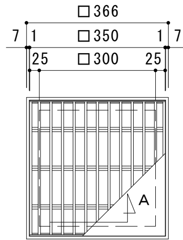
平面詳細図 S = 1 : 10
