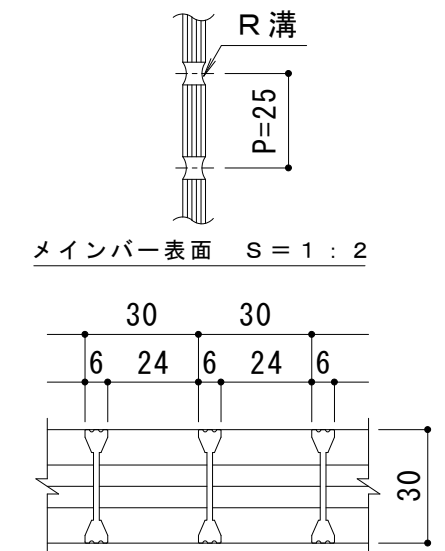
A断面図 S = 1 : 2
