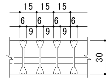
A断面図 S = 1 : 2
