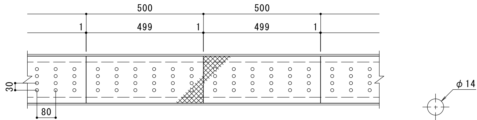
平面詳細図 S = 1 : 10
