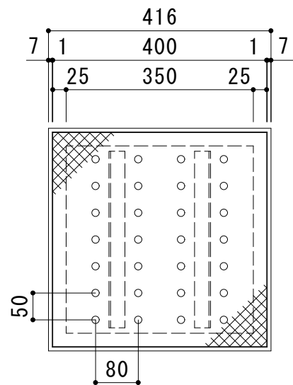
平面詳細図 S = 1 : 10
