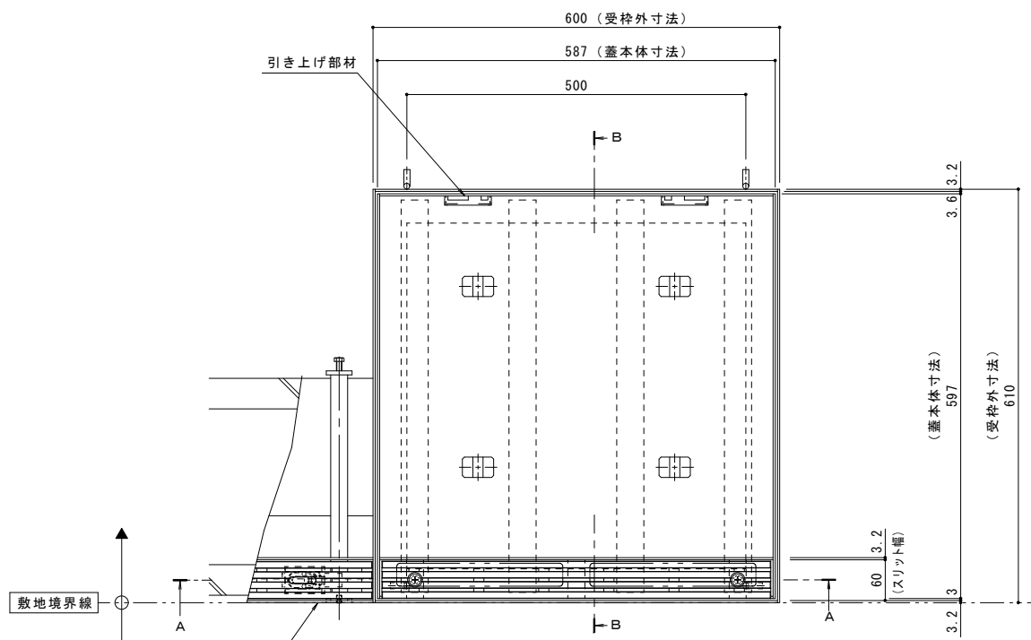
平面図 S=1:5 U字溝用スリットみぞ蓋 集水樹蓋 敷地境界用 VGQM+BKIT
