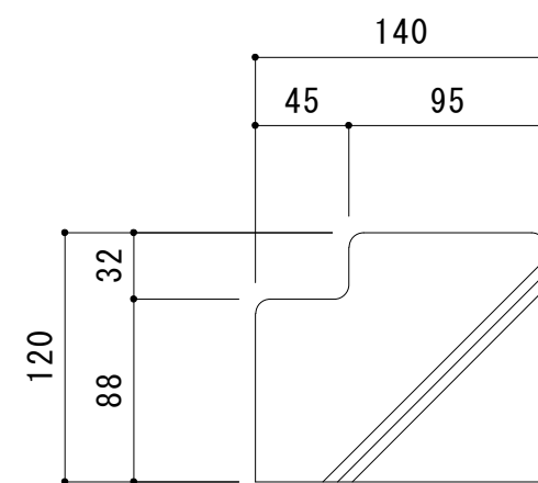
コンクリートブロック断面図 S = 1 : 4
