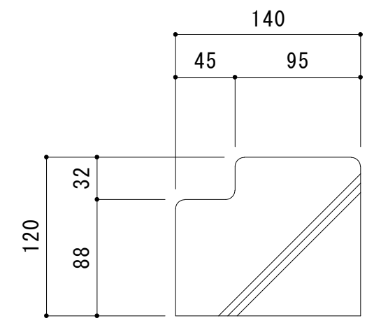
コンクリートブロック断面図 S = 1 : 4
