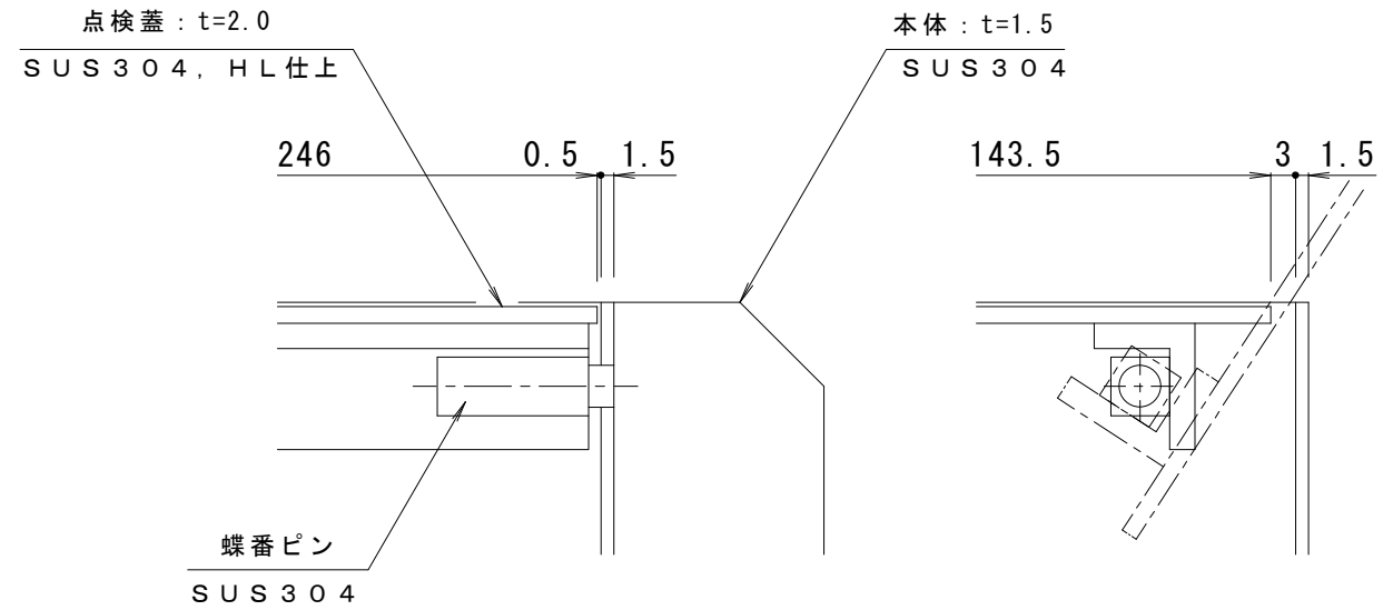
蝶番部 詳細 S = 1 : 1
