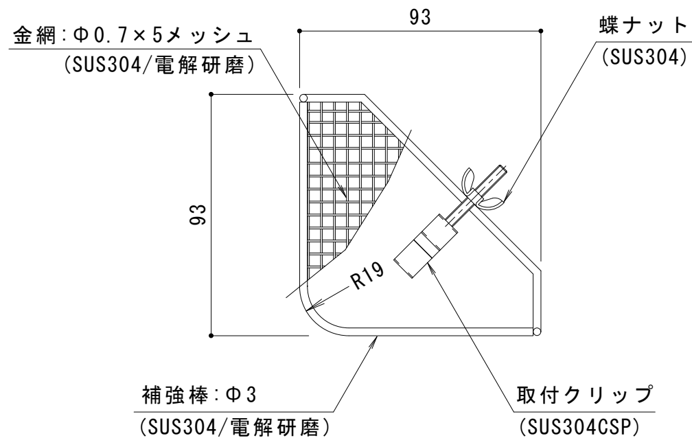
詳細図 S = 1 : 2
