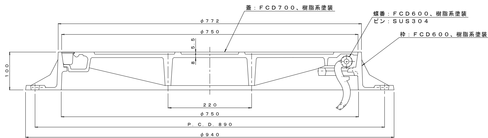
断面 A-A
