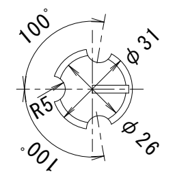
ロックボルト頭部詳細
