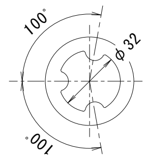
ロック開閉部詳細
