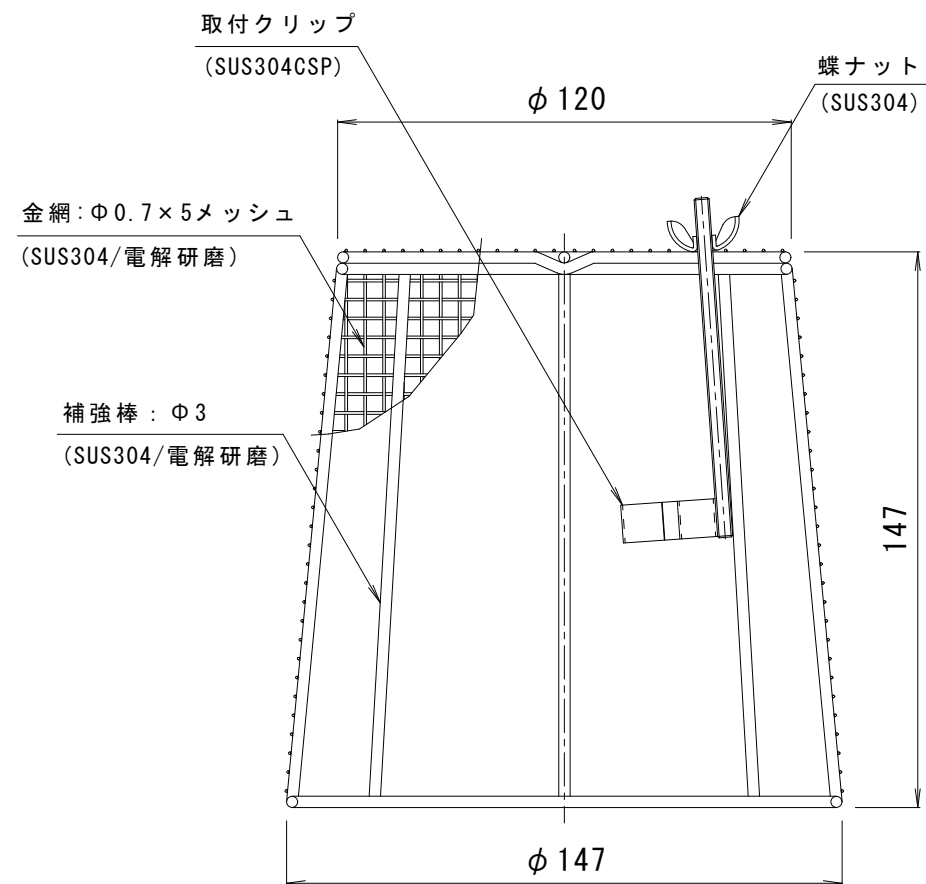
詳細図 S = 1 : 2
