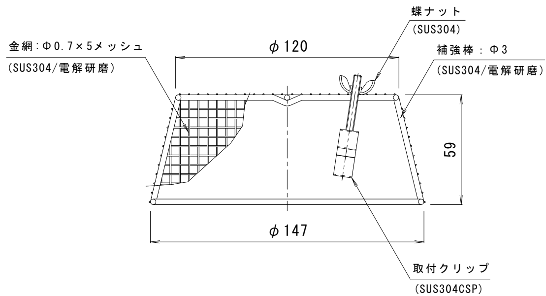
詳細図 S = 1 : 2
