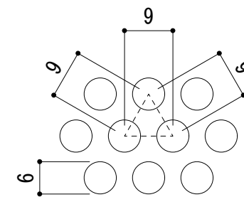
排水穴詳細図 S = 1 : 1
