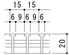
A断面図 S = 1 : 2
