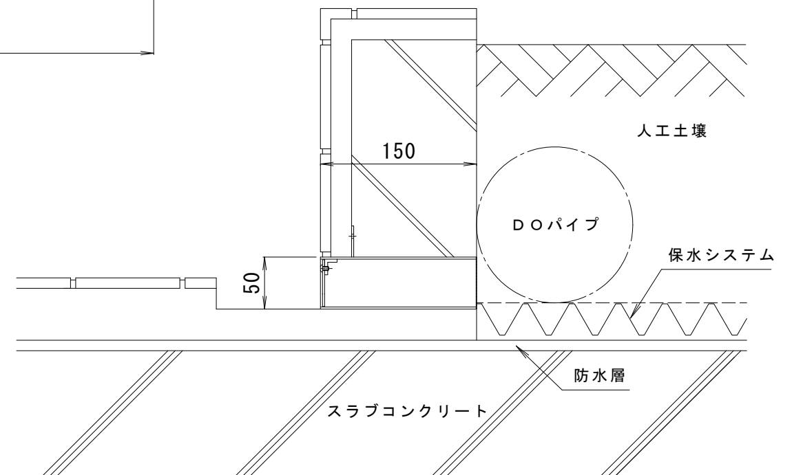
納まり参考図 S = 1 : 5
