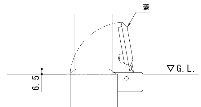
埋設管蓋部詳細図 S = 1 : 3
