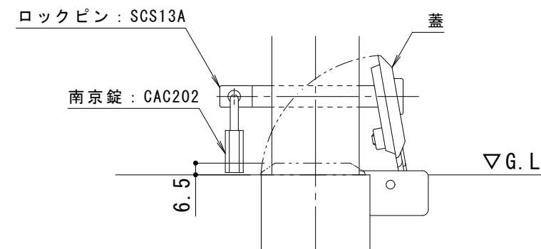
南京錠部詳細図 S = 1 : 3
