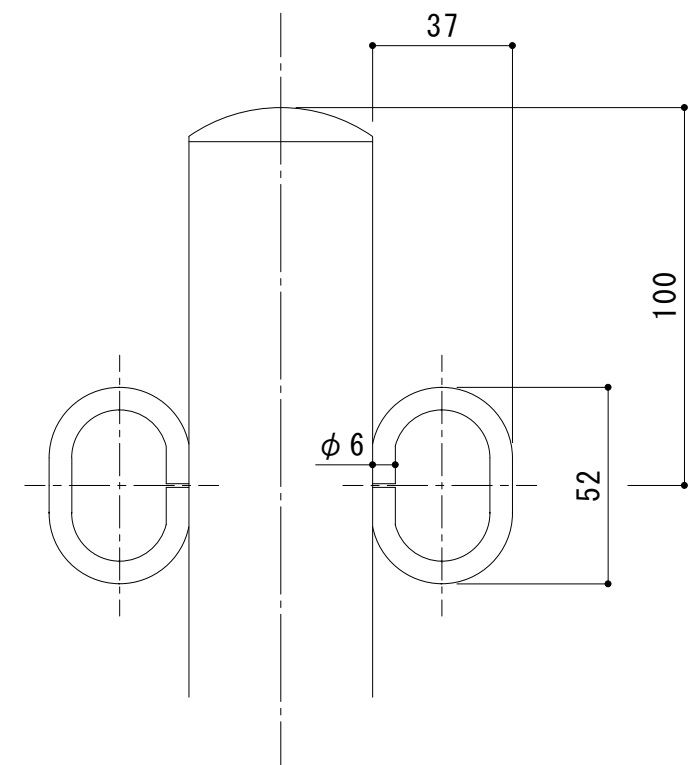
フック部詳細図 S=1:2
