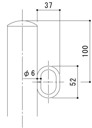
フック部詳細図 S = 1 : 3
