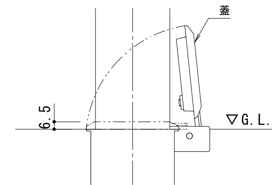
埋設管蓋部詳細図 S = 1 : 3
