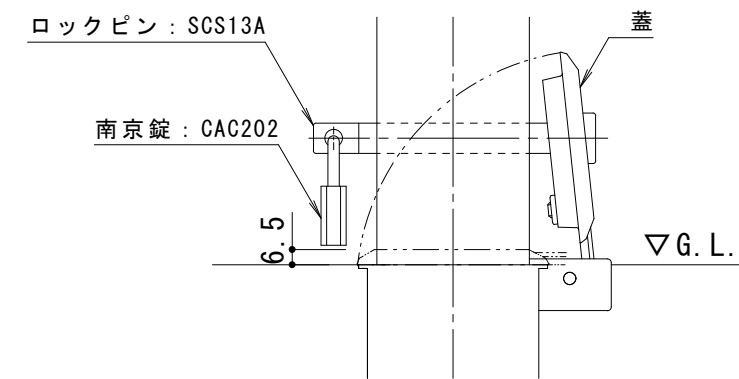
南京錠部詳細図 S = 1 : 3
