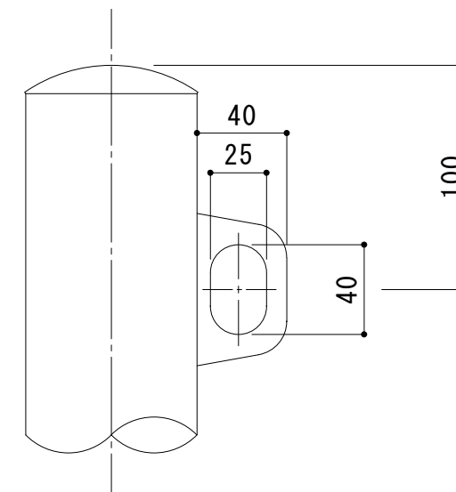
フック部 詳細図 S = 1 : 3
