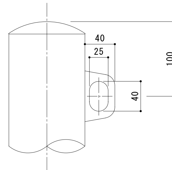
フック部 詳細図 S = 1 : 3
