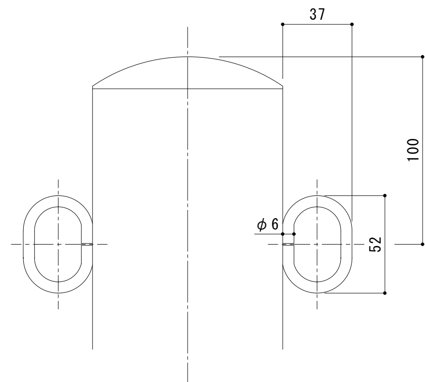
フック部詳細図 S = 1 : 2
