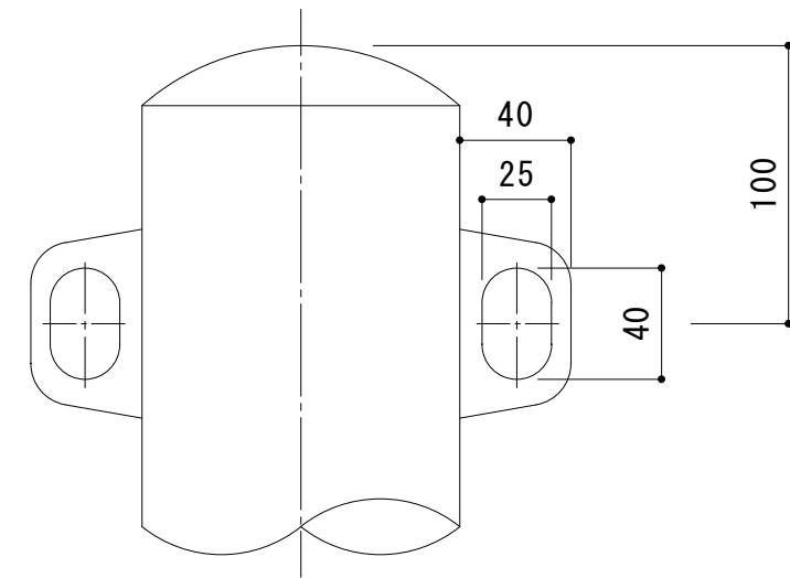
フック部 詳細図 S = 1 : 3
