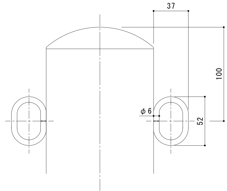
フック部詳細図 S = 1 : 2
