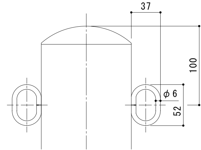
フック部詳細図 S = 1 : 3
