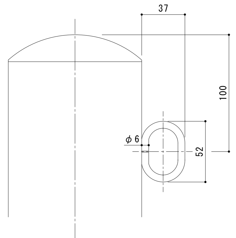
フック部詳細図 S = 1 : 2
