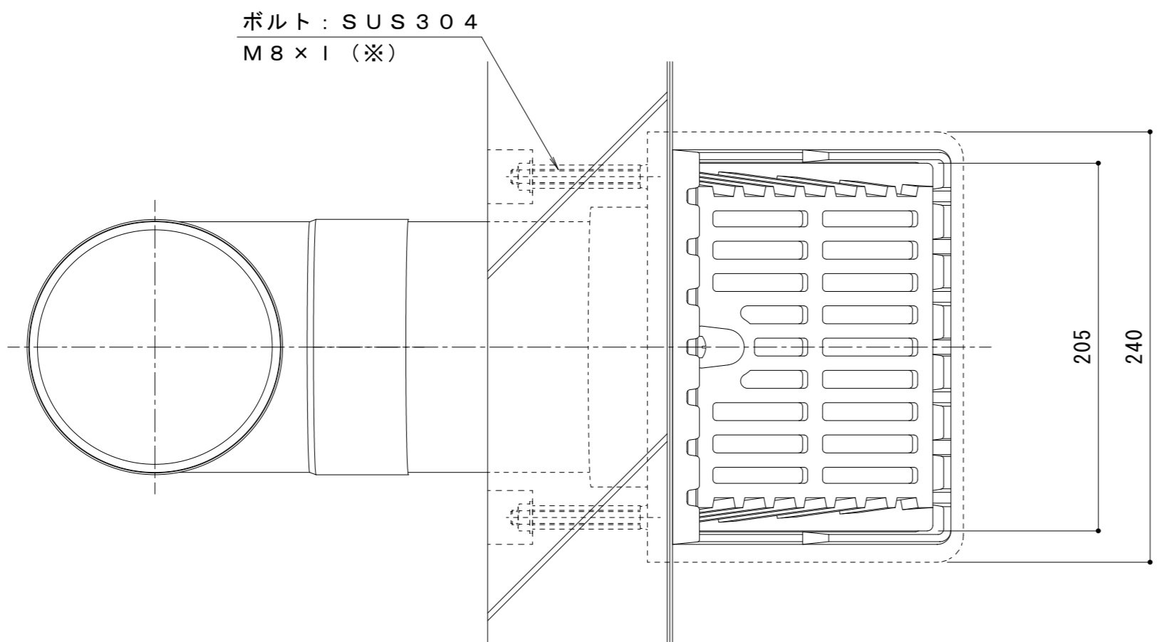
平面図 S = 1 : 3
