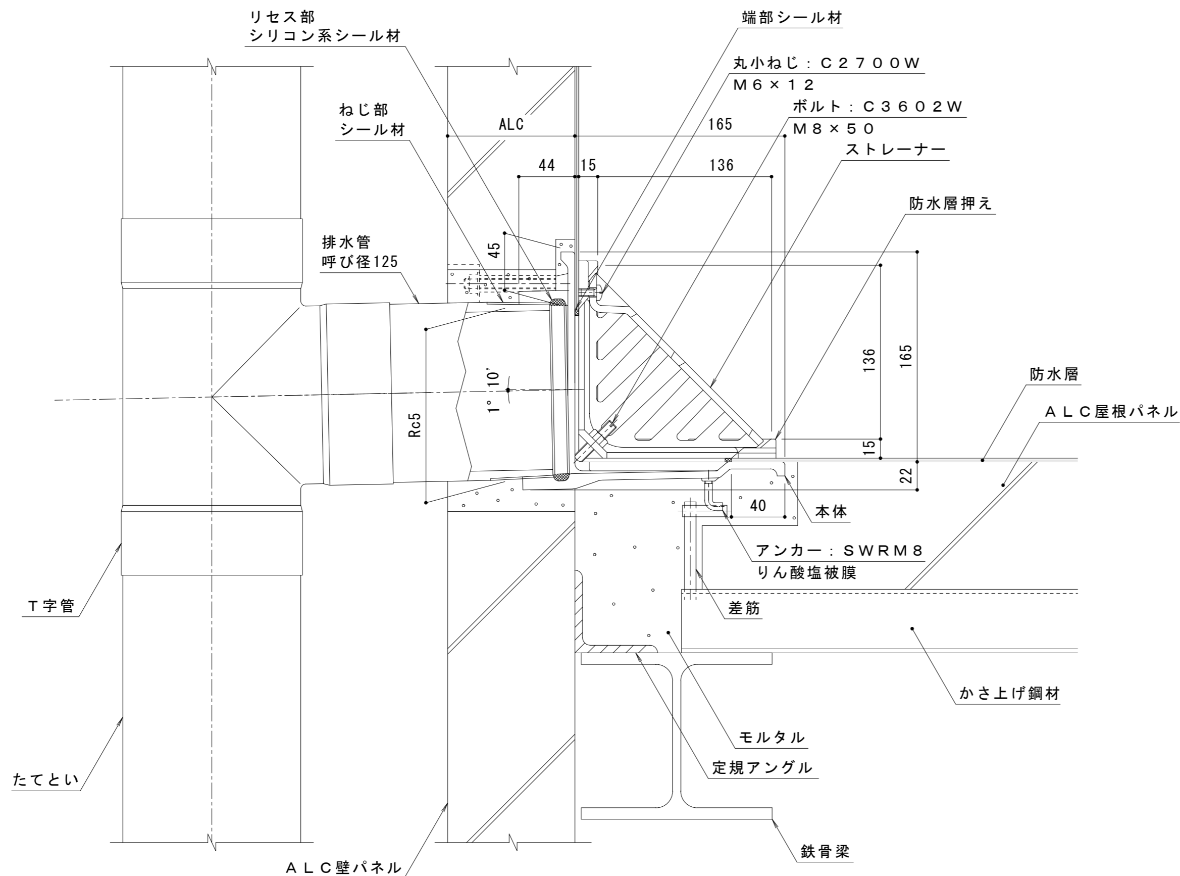
納まり図 S = 1 : 3
