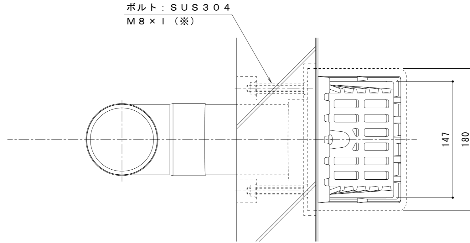
平面図 S = 1 : 3
