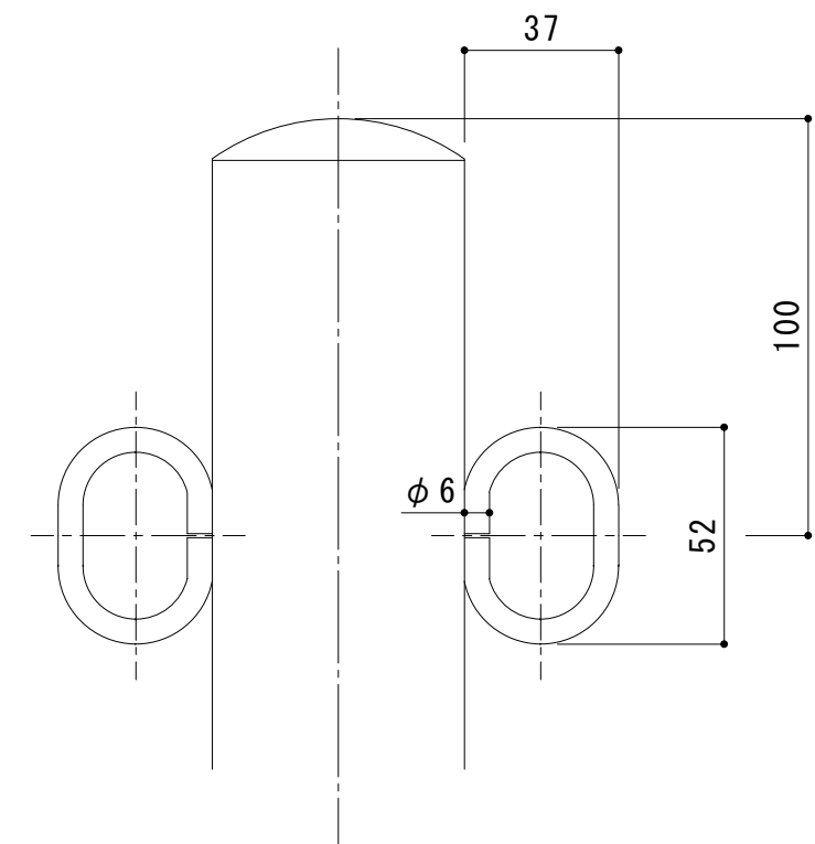
フック部詳細図 S=1:2
