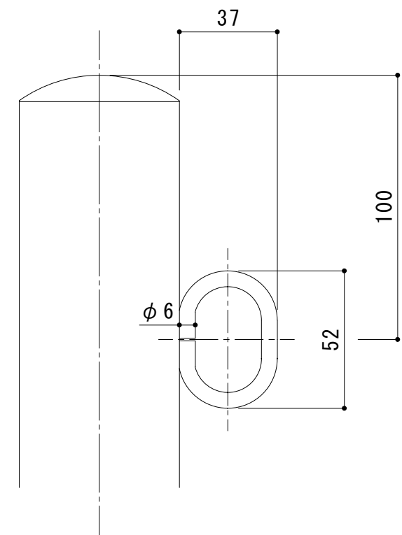
フック部詳細図 S = 1 : 2
