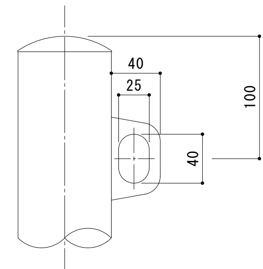
フック部 詳細図 S = 1 : 3
