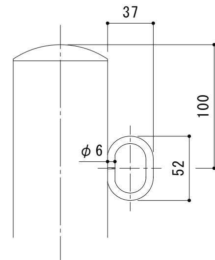
フック部詳細図 S = 1 : 3
