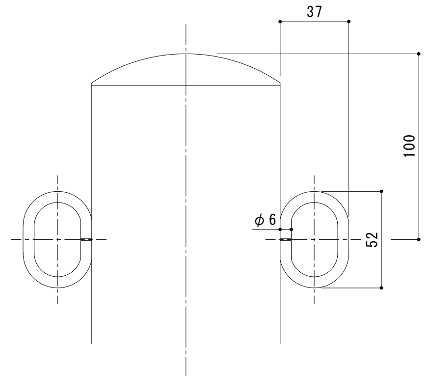
フック部詳細図 S = 1 : 2
