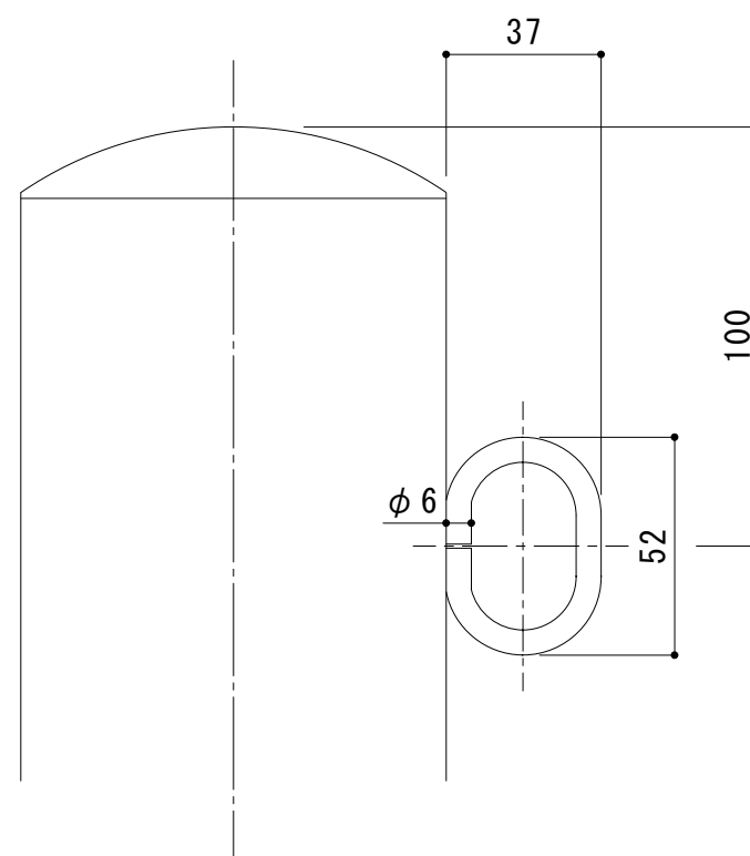
フック部詳細図 S=1:2
