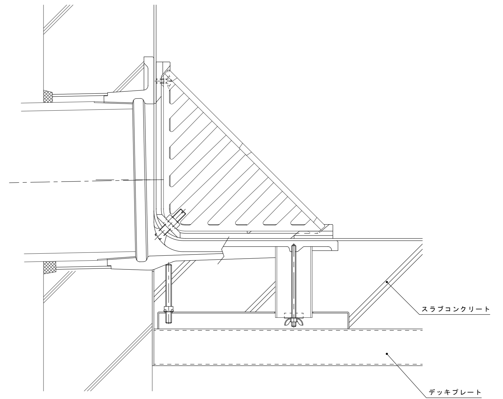
施工例 S=1:3
