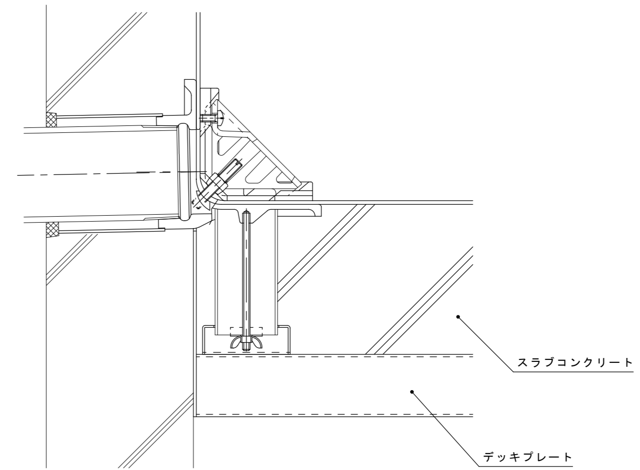
施工例 S = 1 : 3
