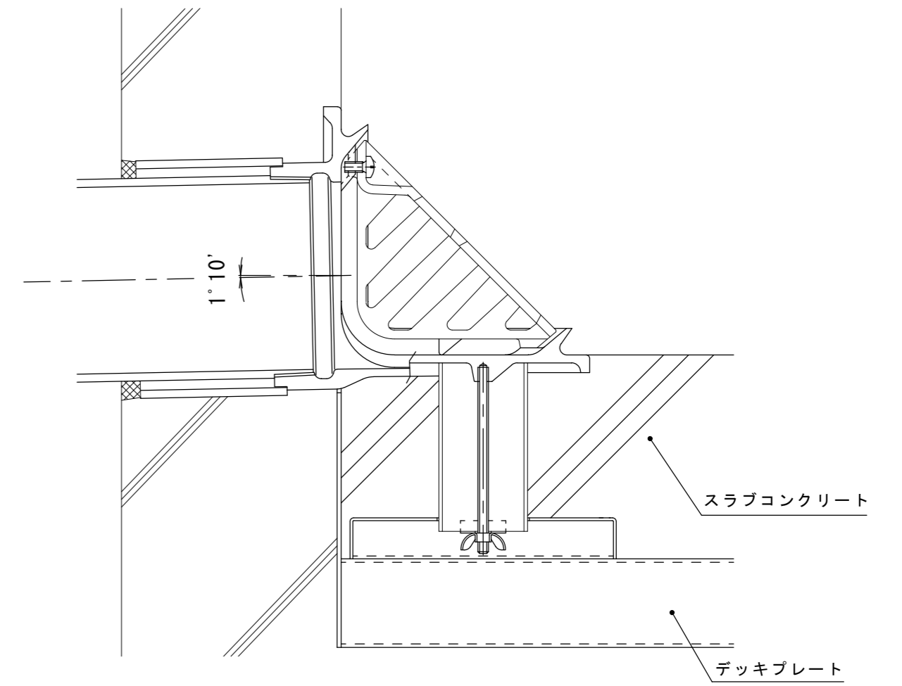
施工例 S = 1 : 3
