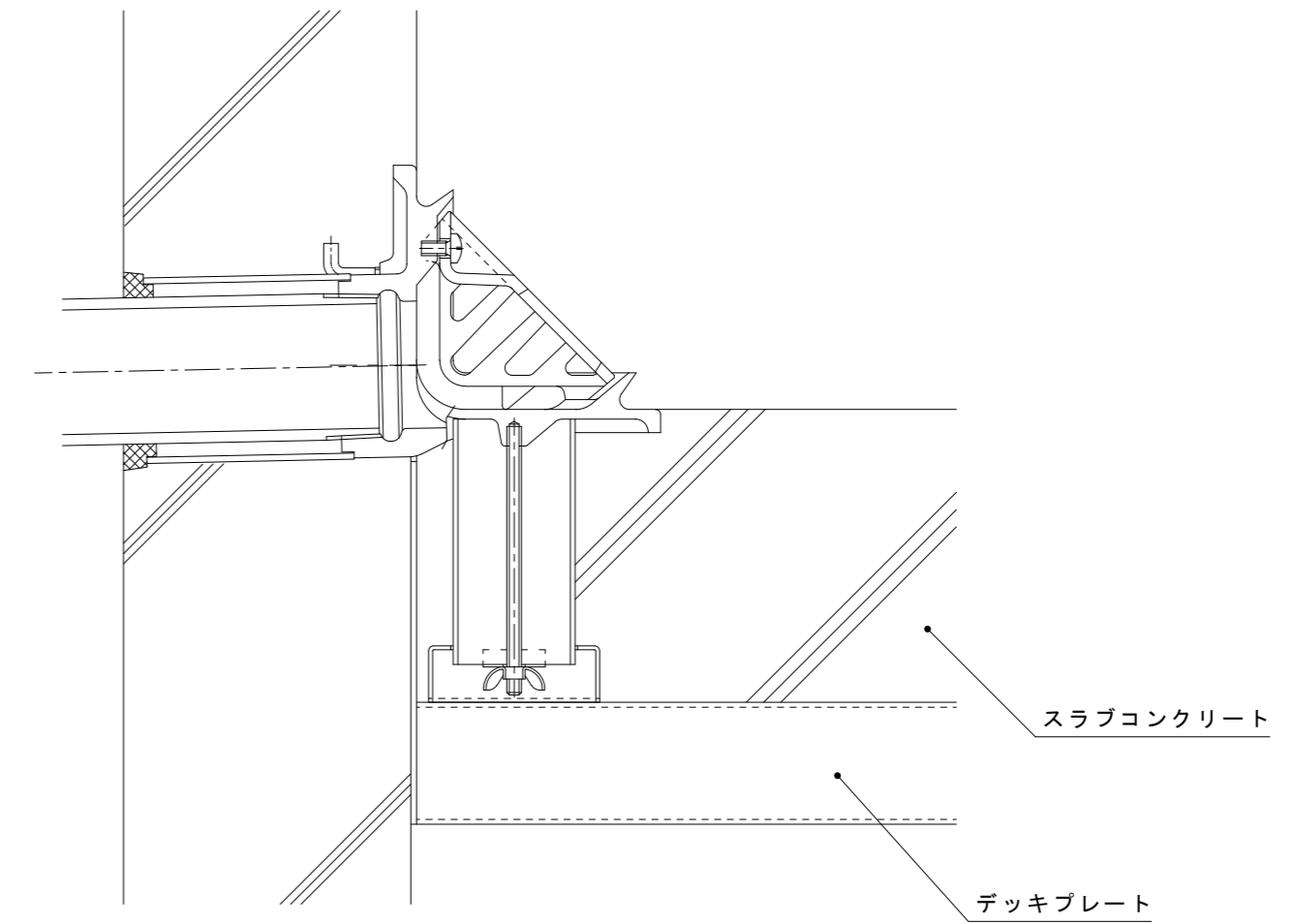
施工例 S = 1 : 3
