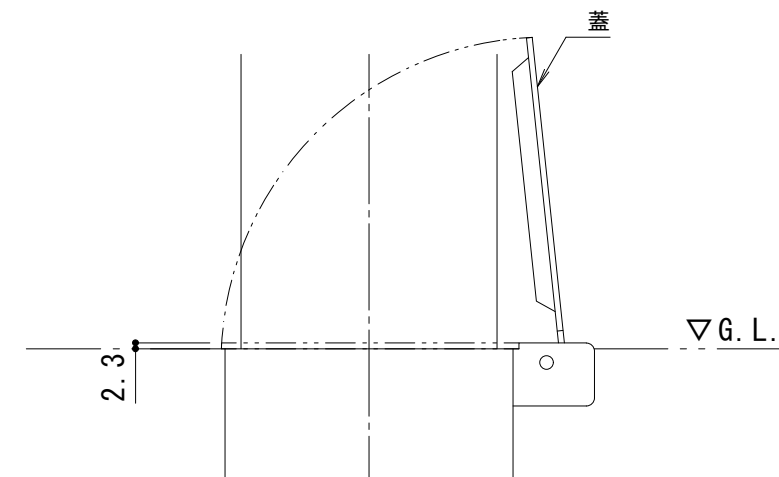
埋設管蓋部詳細図 S = 1 : 3
