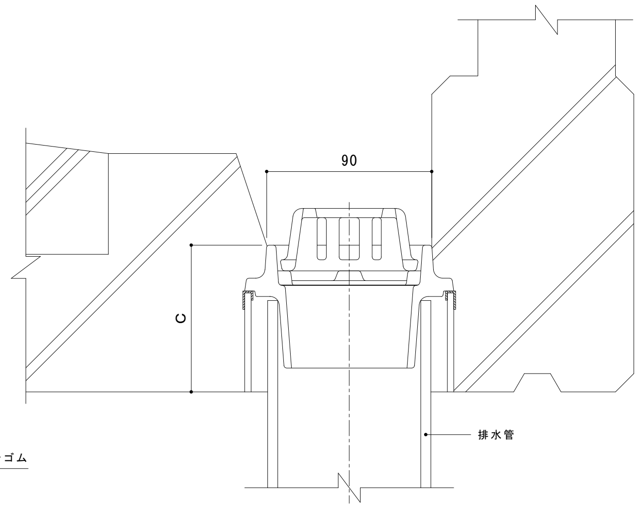
納まり図
