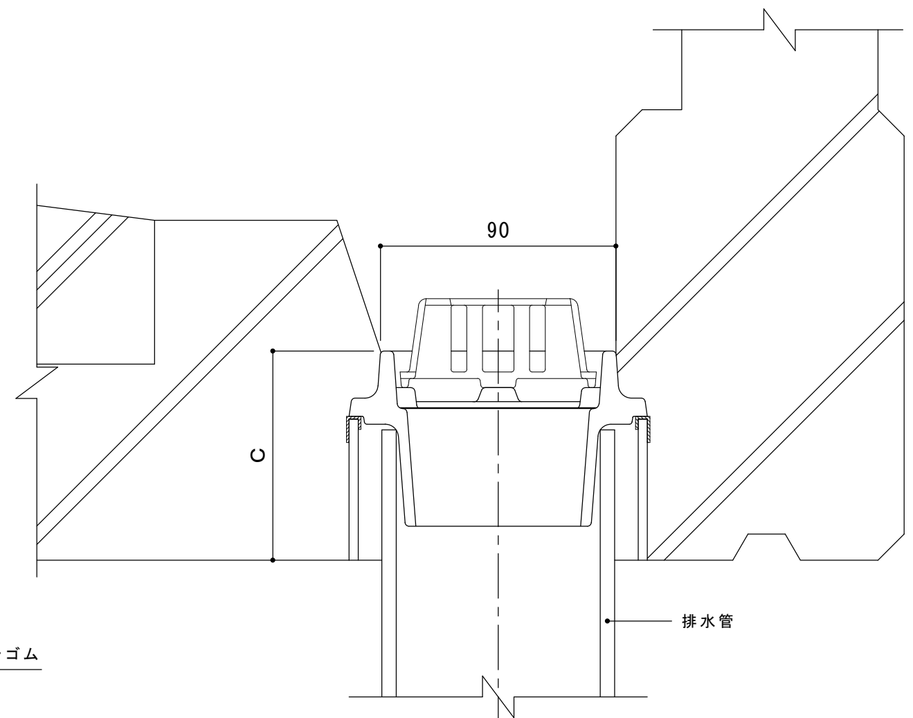
納まり図
