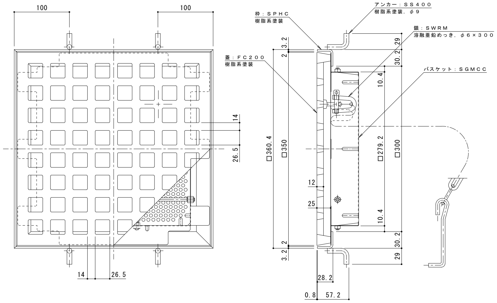
製品詳細図 S = 1 : 3
